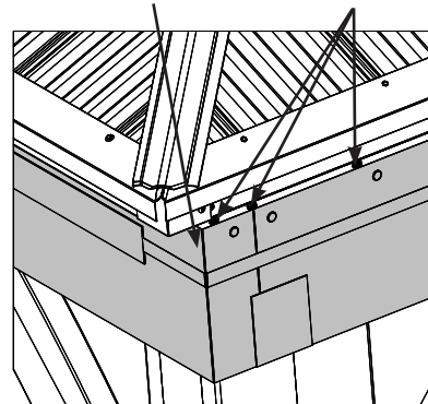
Male Snap with Screw / Broche macho con tornillo / Fixation mâle avec vis
