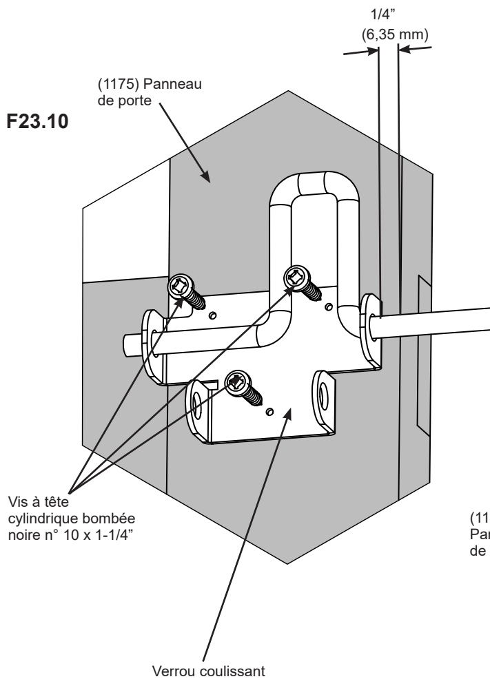
Verrou coulissant
