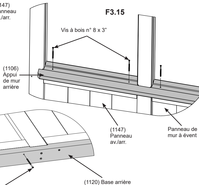
(1147) Panneau av./arr.
